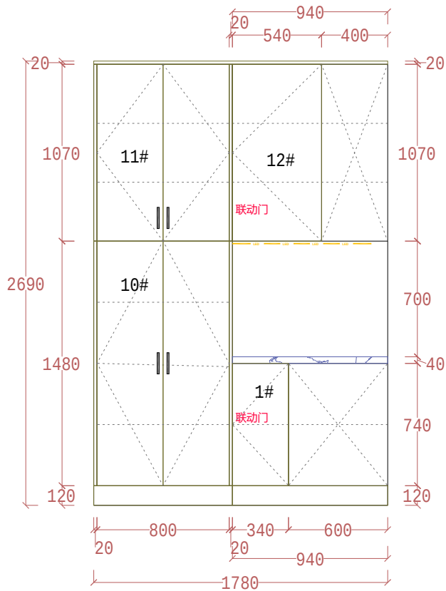
ELEVATION A
