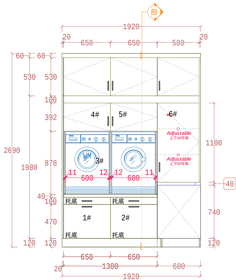
ELEVATION A
