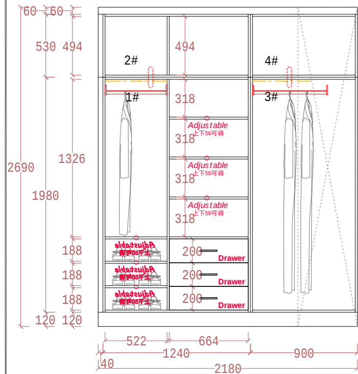
ELEVATION A
