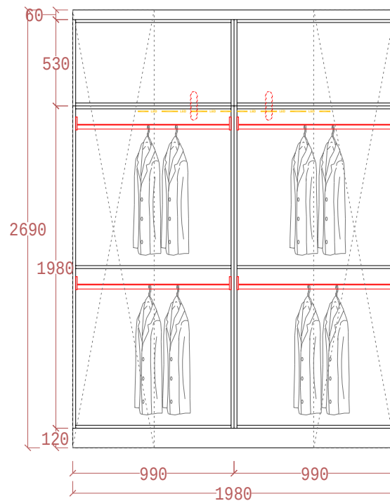
ELEVATION B
