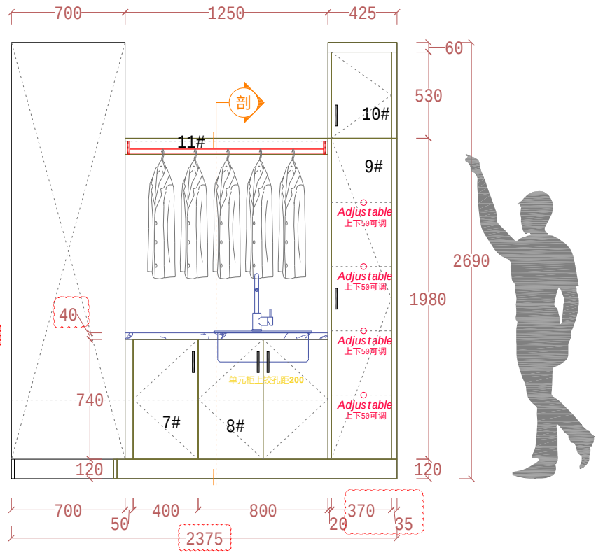
ELEVATION B
