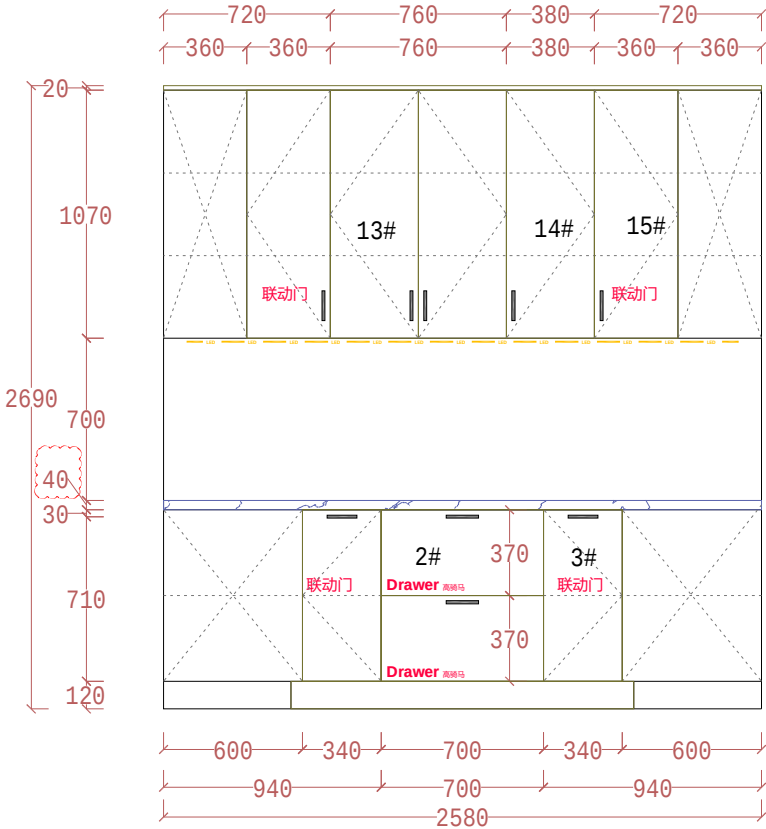
ELEVATION B
